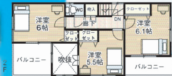
参考プラン例 建延面積/ 92.94㎡(約28.11坪)
