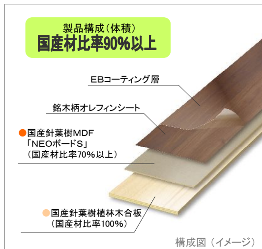
構成図 (イメージ)
