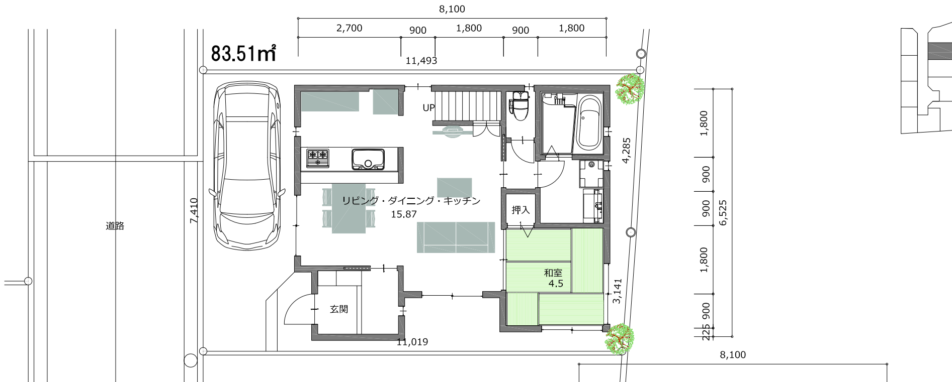
1階平面図
