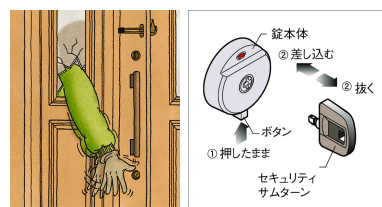
カギがかかっているか確認できるセキュリティサムターン
