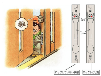
子扉にロック付フランス落としを採用
