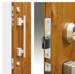
2つの鎌付デッドボルトでこじ開けを徹底ガード
