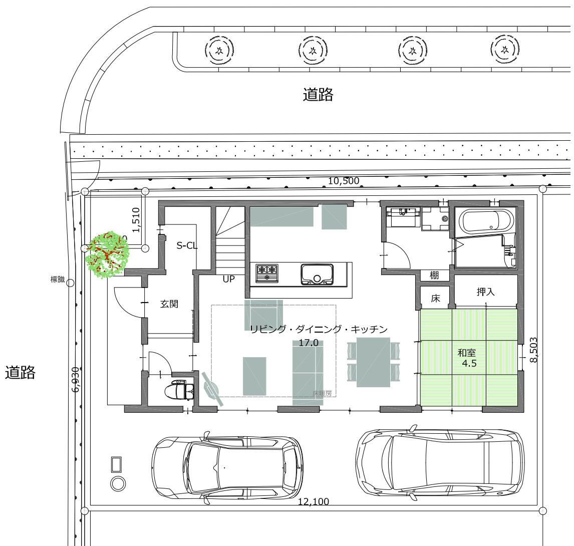
1階平面図
