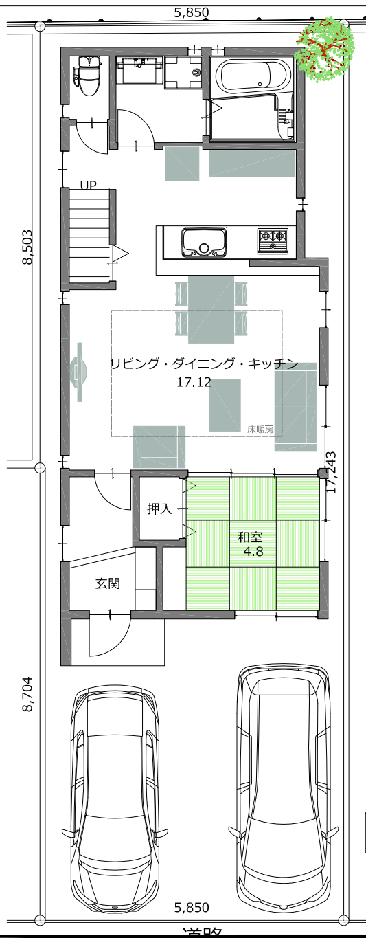
1階平面図
