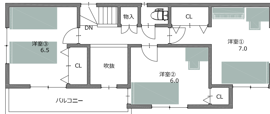
2階平面図
