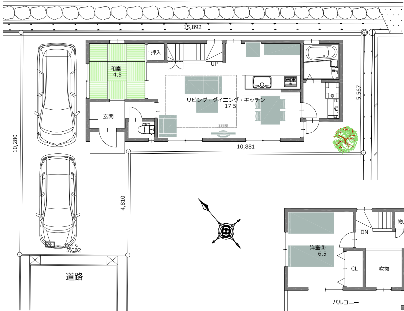
1階平面図
