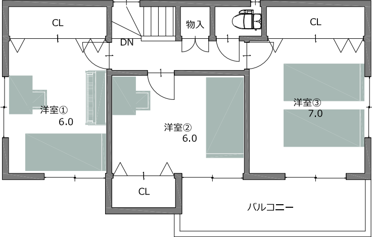
2階平面図
