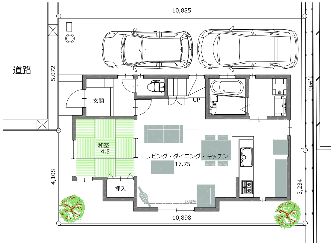
1階平面図
