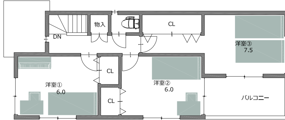
2階平面図
