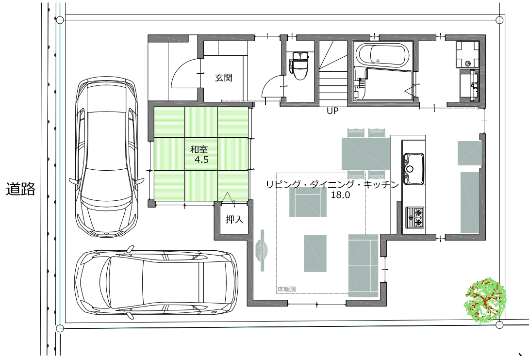
1階平面図
