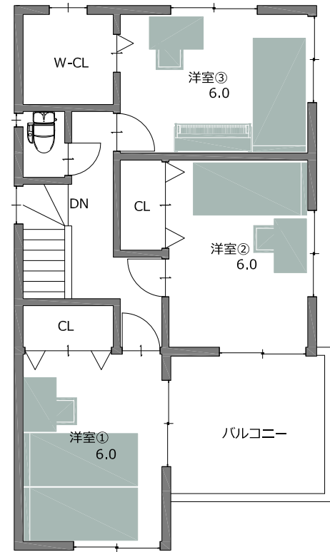
2階平面図
