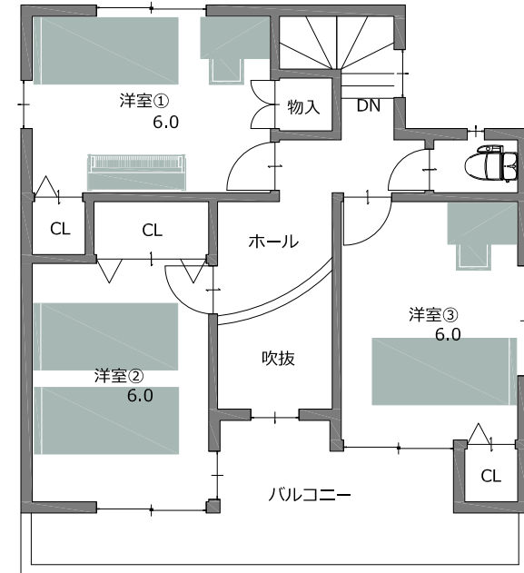
2階平面図
