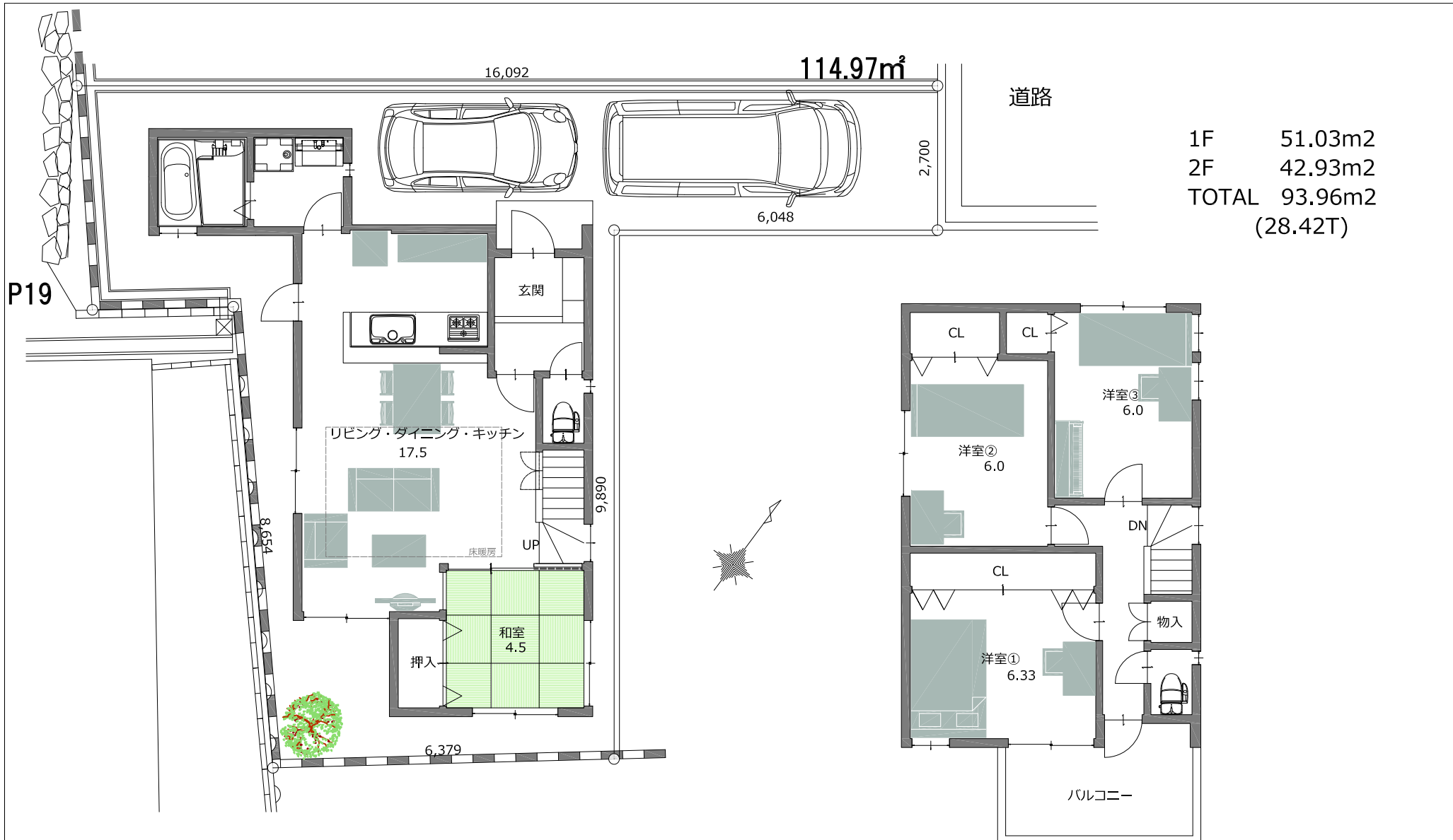
1階平面図
