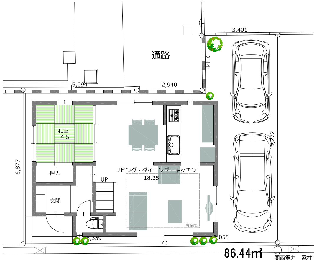
1階平面図
