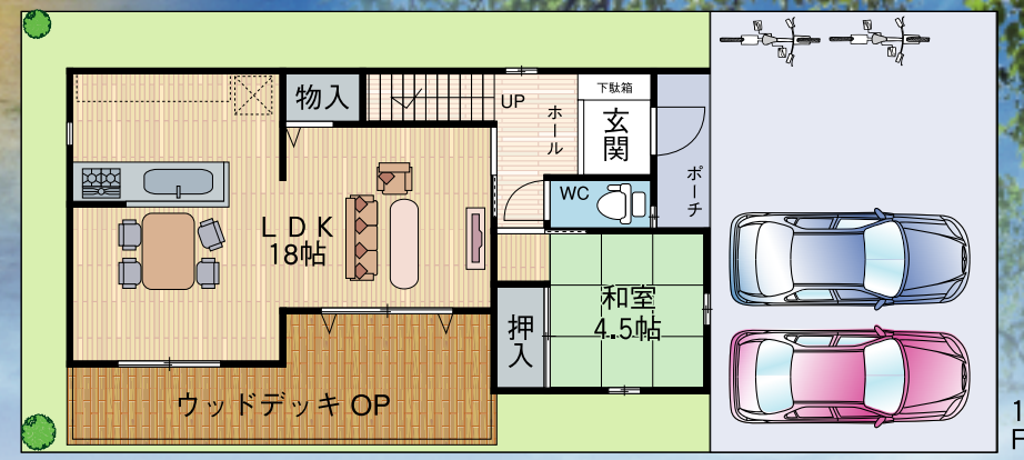
[4号地参考間取りプラン例] 建物参考価格1,300万円(税込) 1階:49.41㎡ 2階:47.38㎡ 延延面積:96.79㎡(29.3坪)
